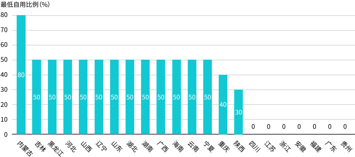
图表 2.10 一般工商业分布式光伏自发自用比例下限
